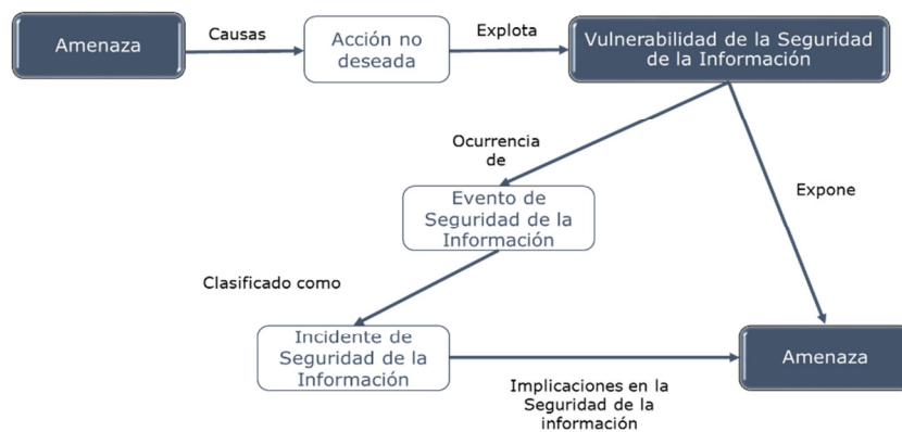
Figura 2. Estructura ISO 27035
